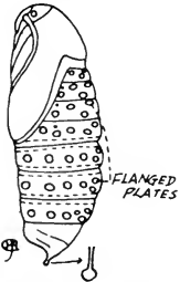
Fig. 525. Isia isabelle S. & A.
